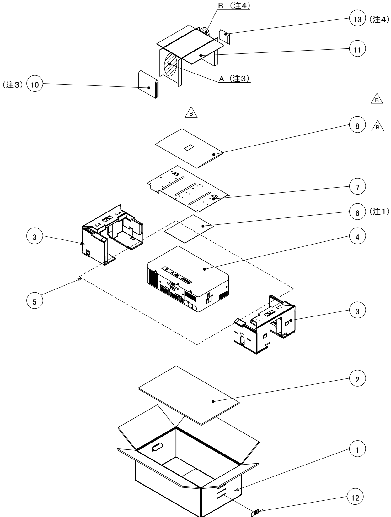
梱包内容説明図(S-Free)
